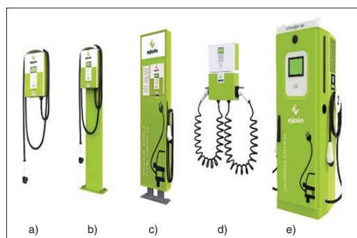
Nabíjecí stanice z produkce ejoin a) nástěnná 22 kW, typ Wallbox, b) sloupek, c) s informačním displejem, d) nástěnná s dvěma nabíjecími místy, e) DC rychlonabíjecí stanice 60/120kW
